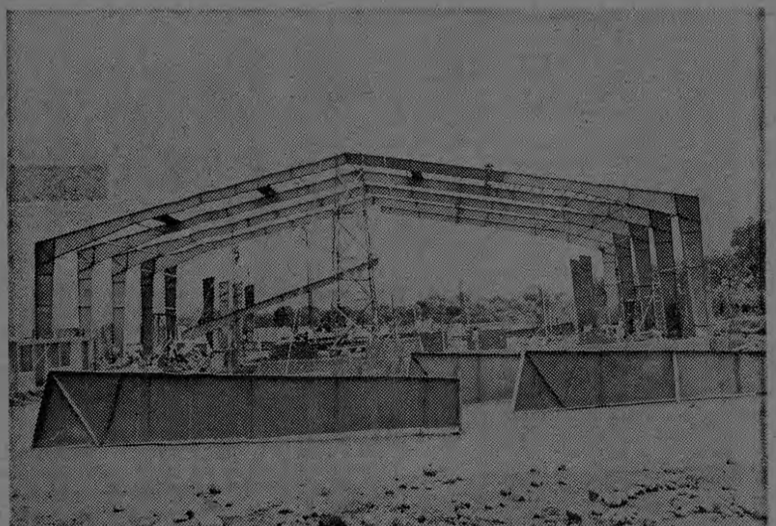
Estructura de marcos rígidos de ACERO en ALMA LLENA, en ejecución por PANEFOM S. A., y la firma Inspector AICA SACMAG. Tiene un claro de 52 metros, fondo 102 metros, altura de cumbrera 14.5 metros, AREA 5,304 m 2 . Será un Depósito más para ALMACEN CENTRAL DE DEPOSITOS S. A. Es la estructura mayor, en su género, construida en Costa Rica.
